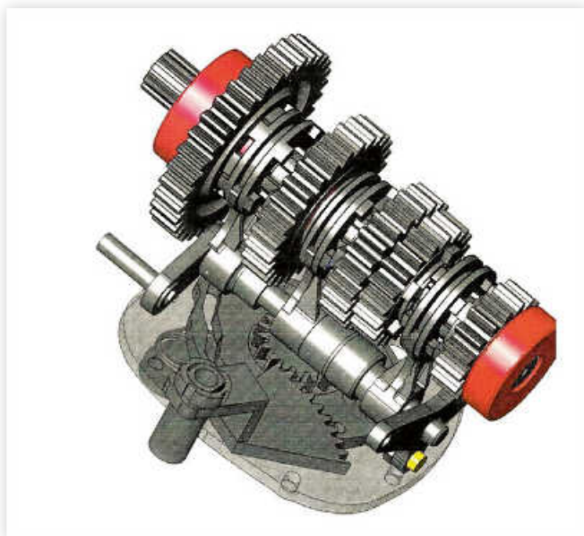
Getriebe 5-Gang
