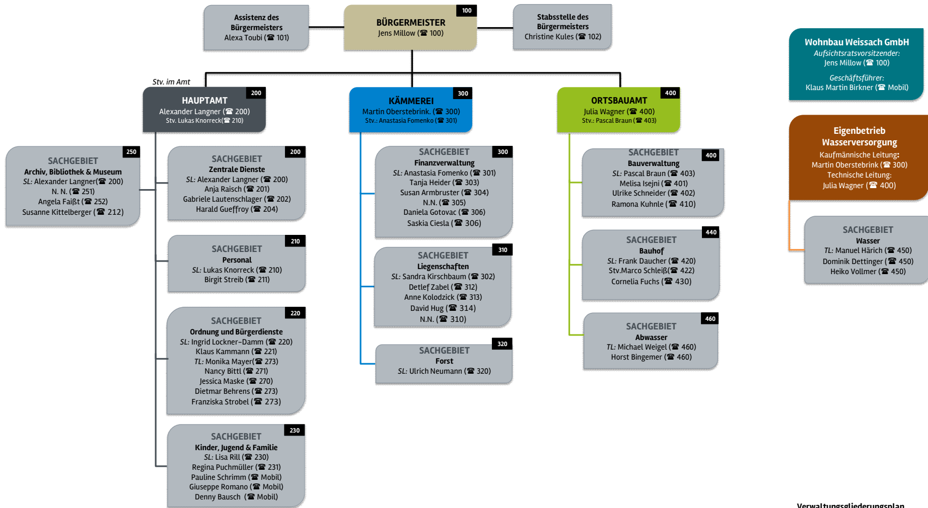
Verwaltungsgliederungsplan (Aufbauorganisation)
